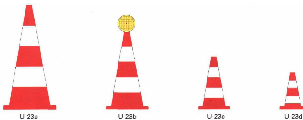
Rys. 9. Wzory pachółków drogowych U-23
