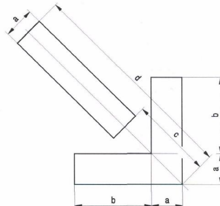
Rys. 19. Geometria strzały świetlnej na tablicy zamykającej U-26
